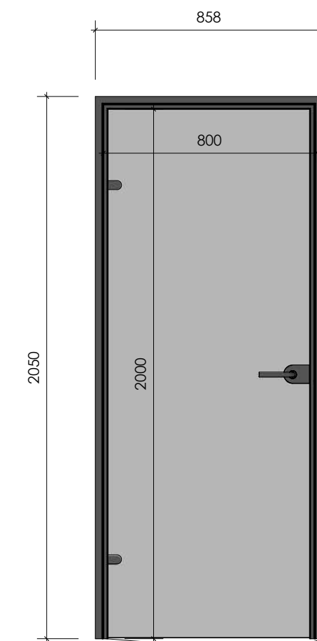
Стеклянная дверь с алюминиевой рамой
