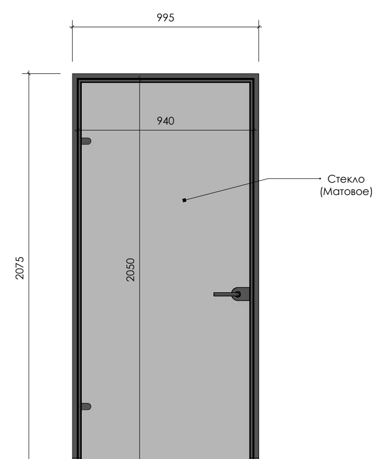
Стеклянная дверь с алюминиевой рамой
