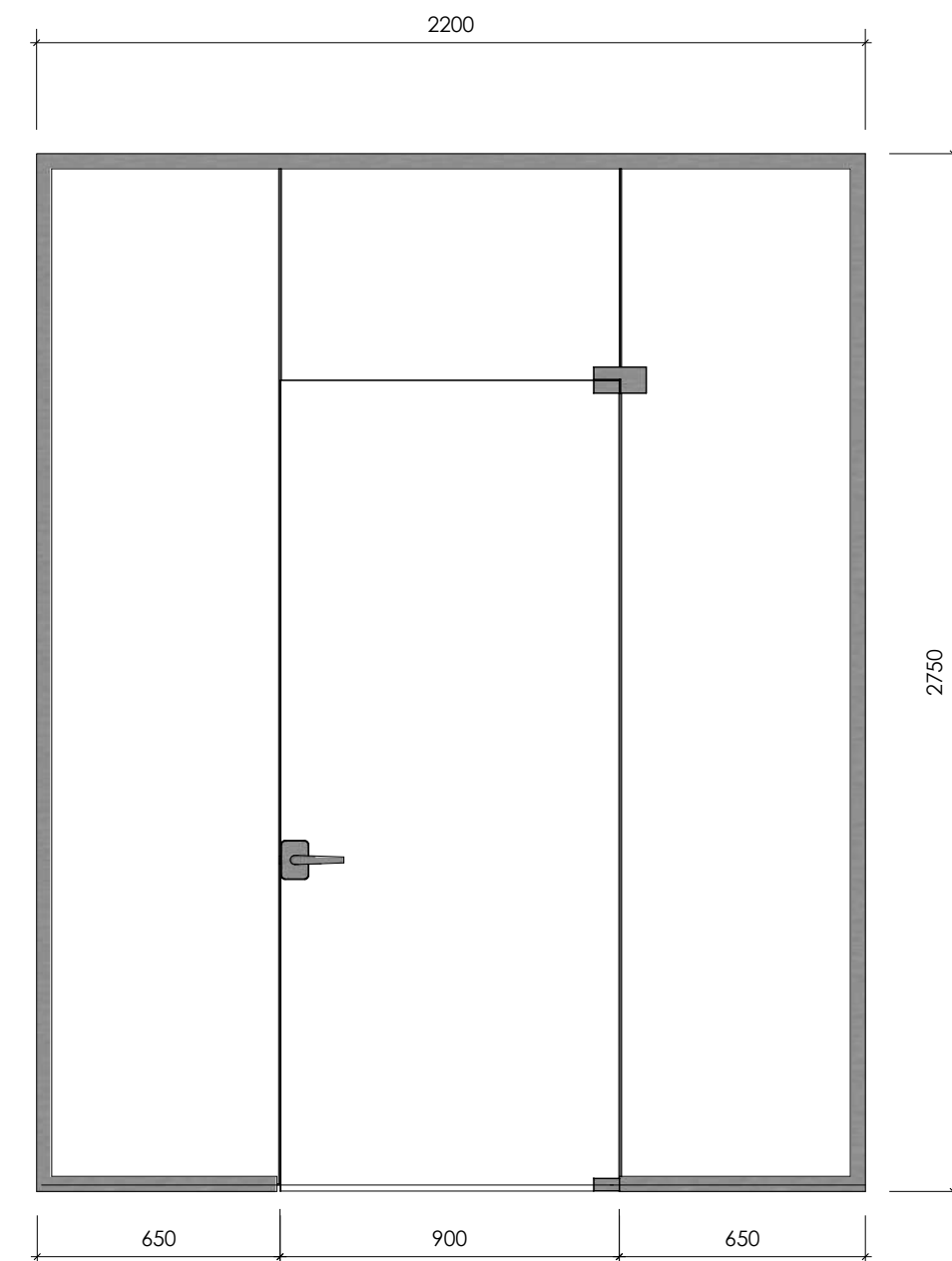
Дверь с перегородкой из монолитного стекла (администраторская)
