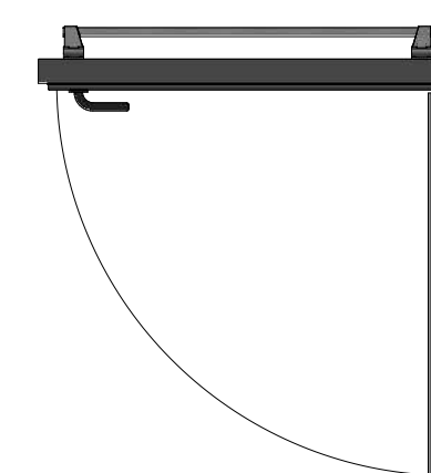
Противопожарная дверь с ручкой "антипаника"
