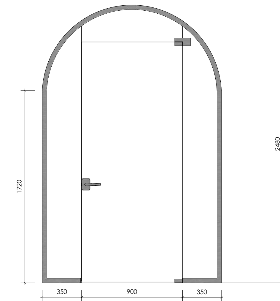
Дверь с перегородкой из монолитного каленного стекла
