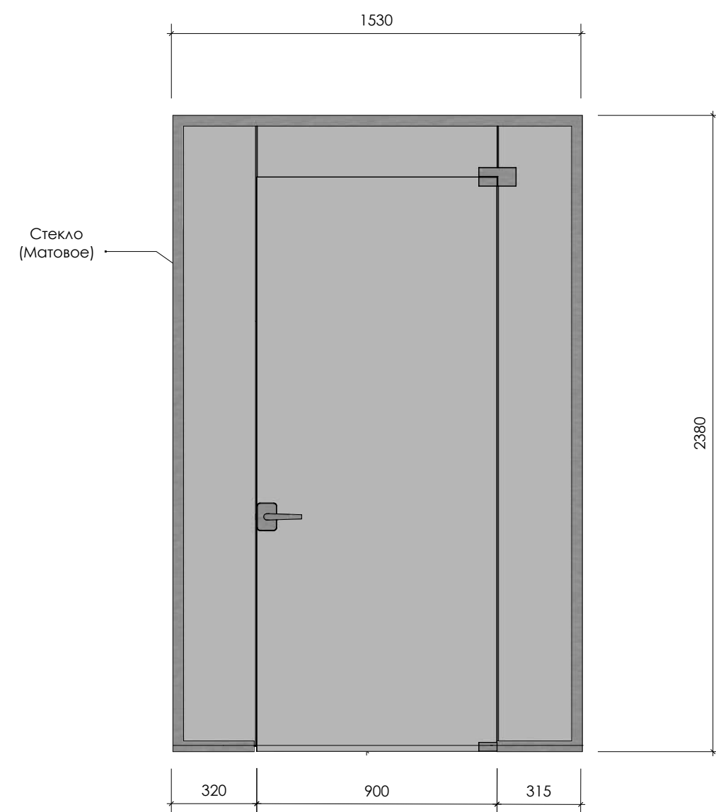
Дверь с перегородкой из монолитного стекла
