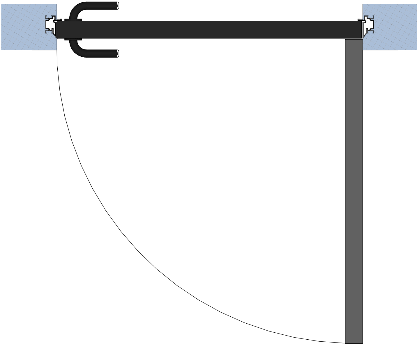
Дверь скрытого монтажа с покраской в цвет стены
