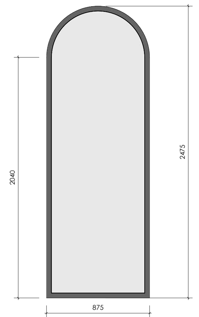
Стеклопанель перегородка без двери
